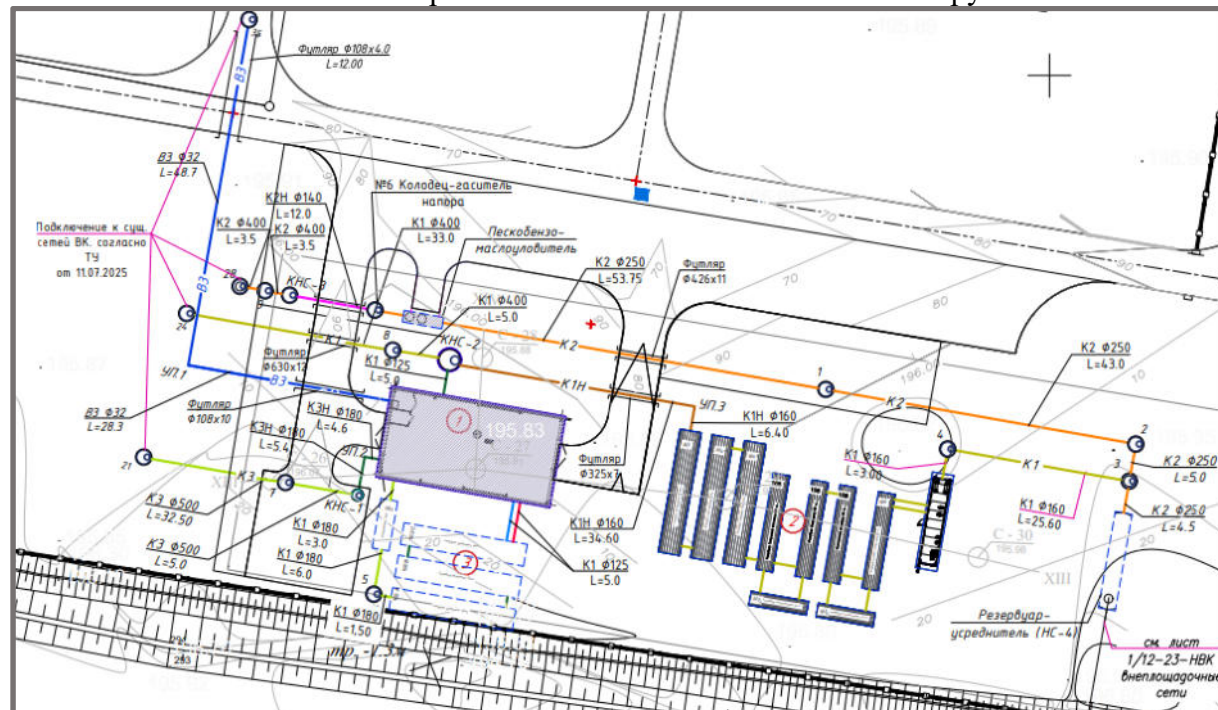
План расположения объектов очистных сооружений
