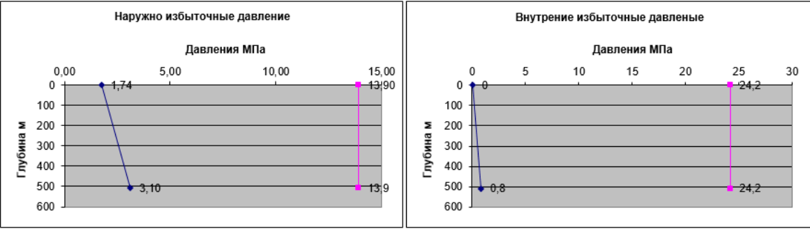
Рисунок 9.1-Распределение избыточных давлений (кондуктор)
