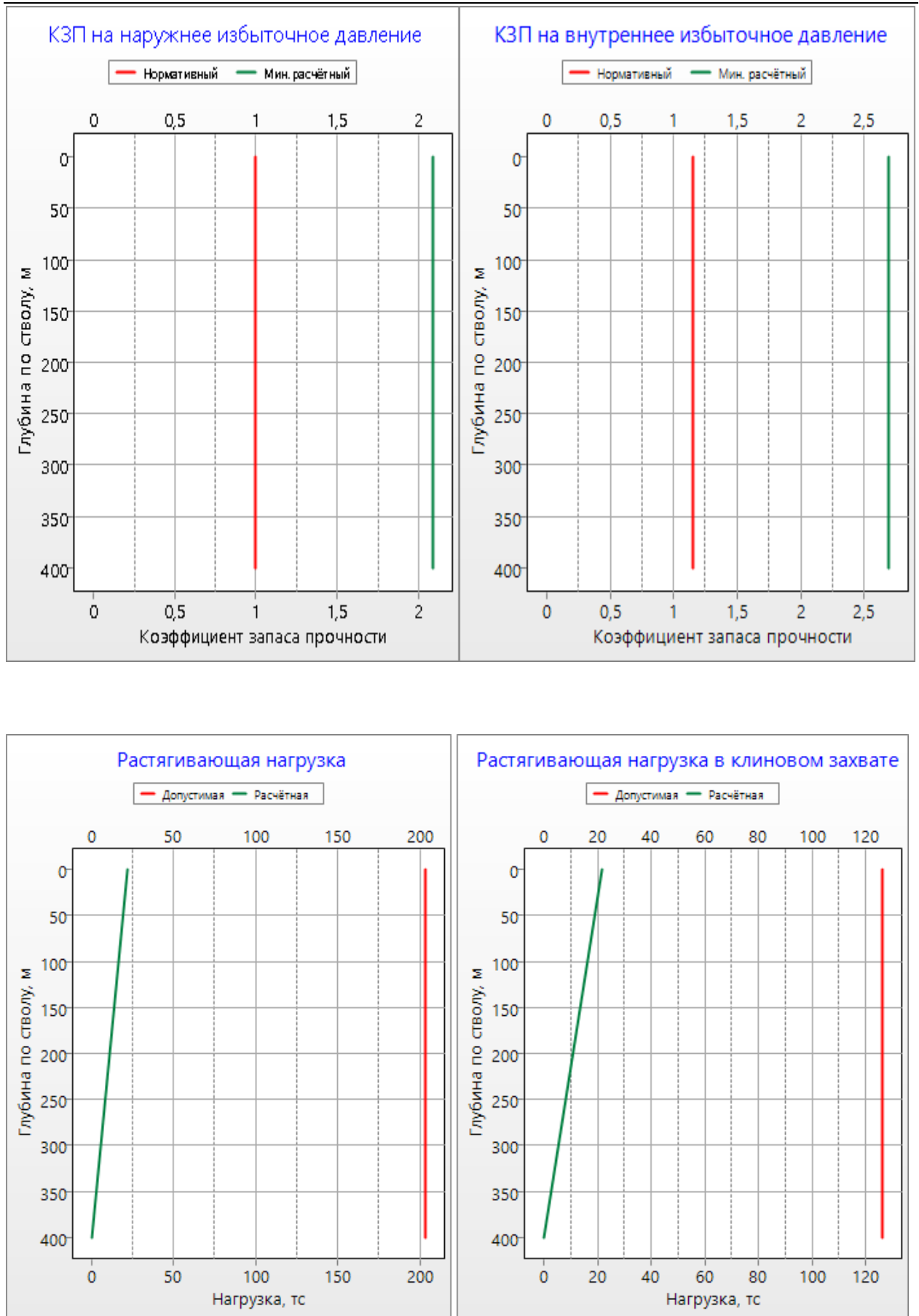
Рис. 9.1 - Эпюры избыточных давлений для колонны диаметром Ø244,5мм
