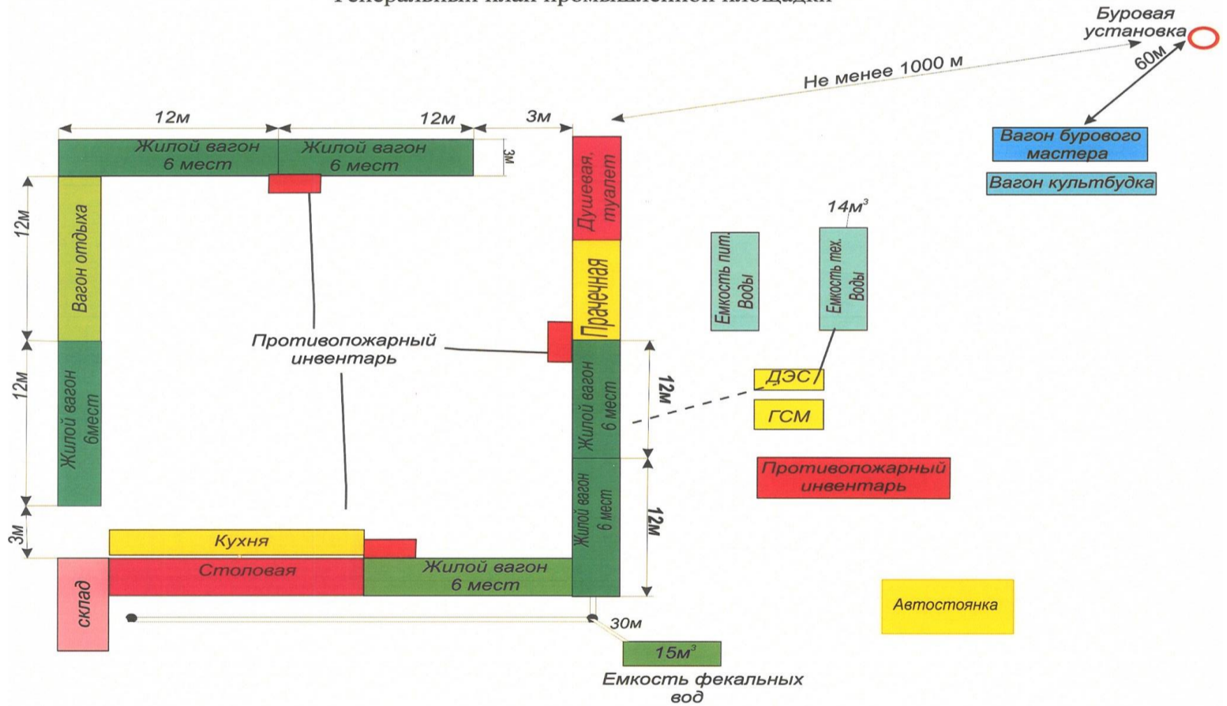
Генеральный план промышленной площадки
