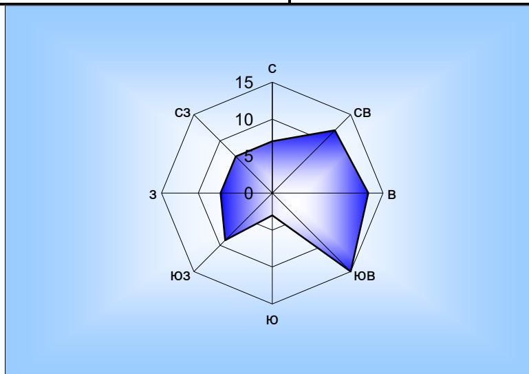
Рисунок 1.1. Роза ветров Кызылкогинского района
