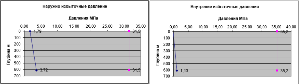
Рисунок 9.1-Распределение избыточных давлений (эксплуатационная колонна)
