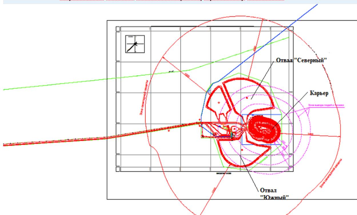
Схема расположения объектов рудника Жуантобе Жуантөбе кеніші объектілерінің орналасу схемасы
