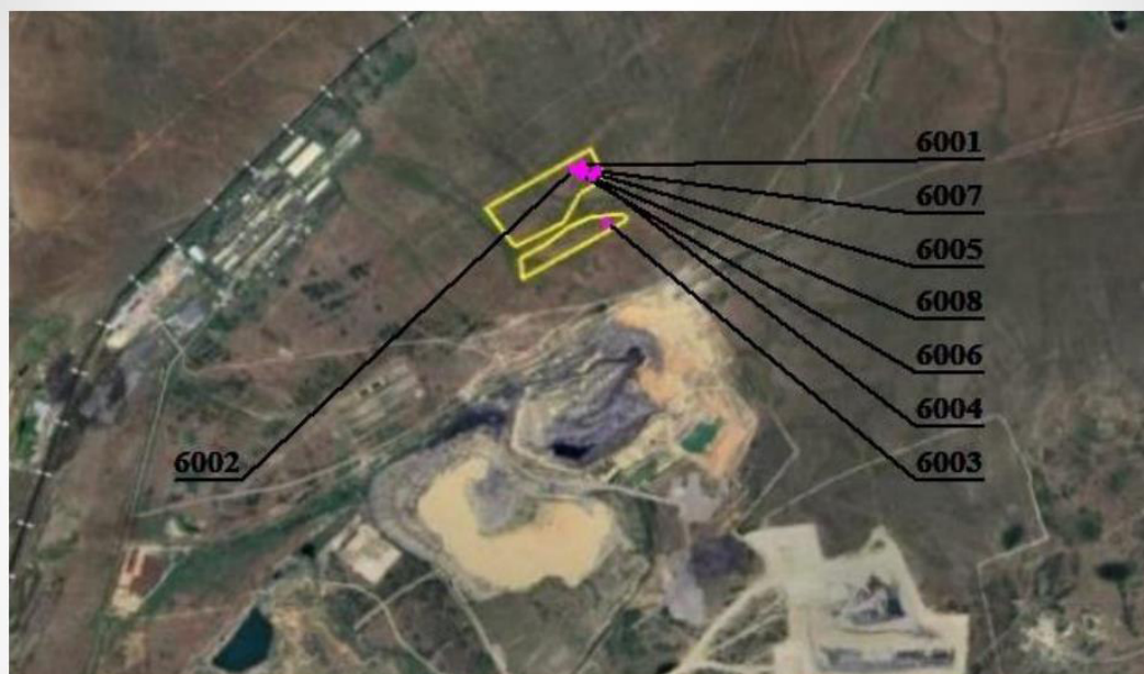
Шығарындылар көздерінің өнеркәсіптік алаңда орналасуы Расположение источников выбросов на промплощадке
