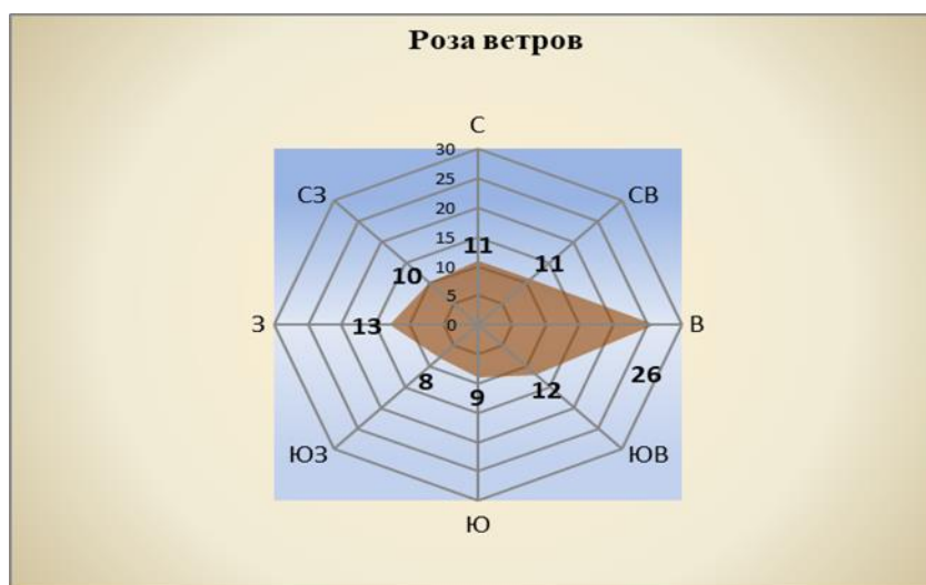
Рисунок 3.1 - Роза ветров
