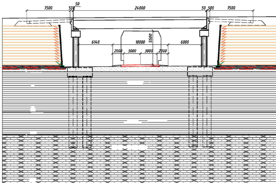
Фасад М 1:200
