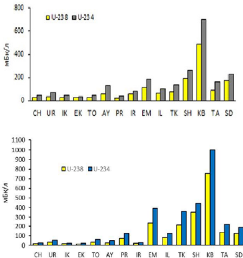
Рисунок 3.6 Результаты радиохимического анализа проб воды, отобранных в бассейнах трансграничных рек Казахстана весной (вверху) и осенью (внизу) 2020 года
